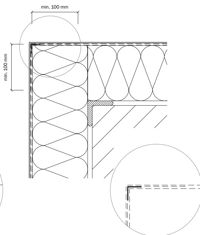
b) Võrguga nurgaprofiil. Lahendus topeltarmeeringu korral
