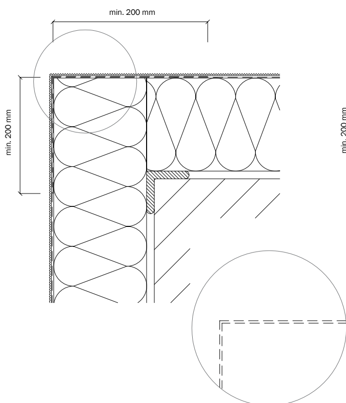
c) Armeerimisvõrguga nurga vormistamine
