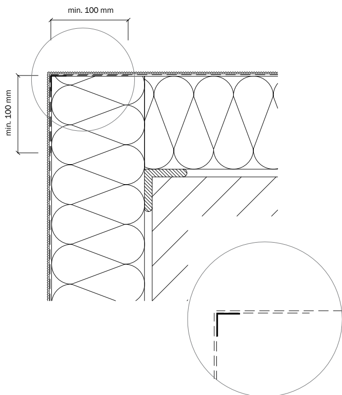
a) Võrguga nurgaprofiil
