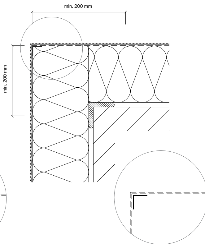
d) Võrguga nurgaprofiil
